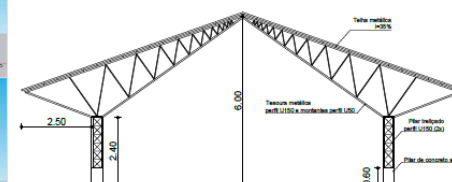
CORTE TRANSVERSAL
